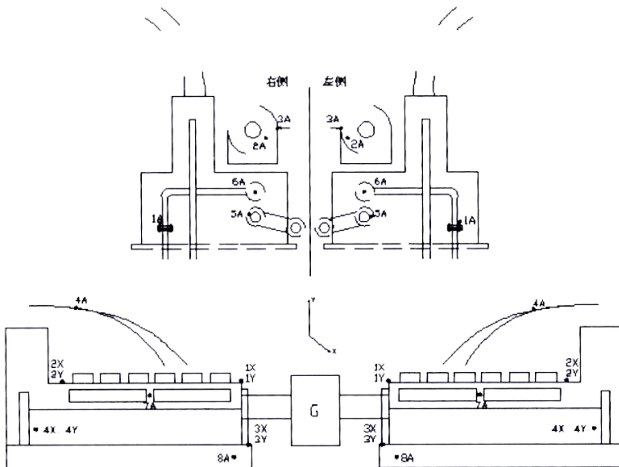
(1核) 振动测点布置图
